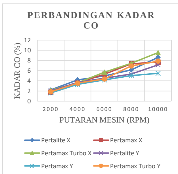
Gambar 14. Grafik perbandingan kedua kadar CO
