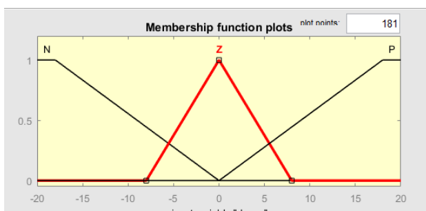
Gambar 6. Membership function untuk input delta error
