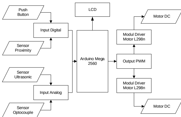
Gambar 2. Diagram alir sistem AGV
