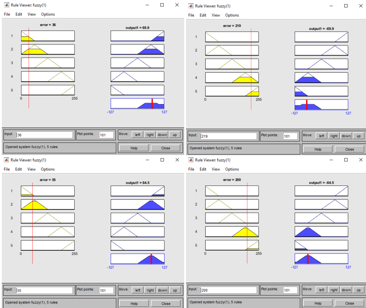
Gambar 11. Sampling hasil nilai output fuzzy dari beberapa nilai input (error) yang berkorelasi pada nilai positif dan negative
