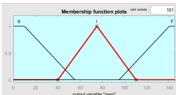
Gambar 7. Membership function untuk output pulsa pwm Nilai pada input membership function
