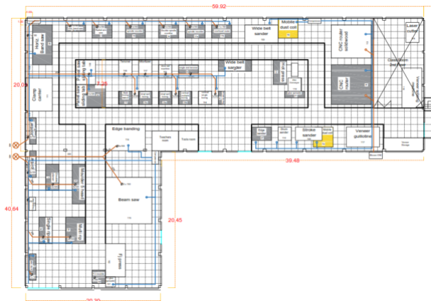
Gambar 3. Denah Workshop Furnitur Politeknik Industri Furnitur dan Pengolahan Kayu
