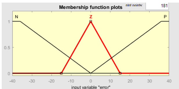
Gambar 5. Membership function untuk input error
