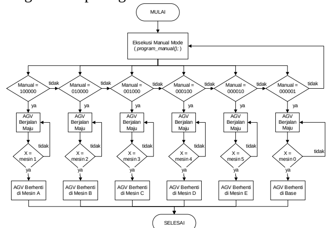
Gambar 4. Diagram Alir Sistem Gerak AGV
