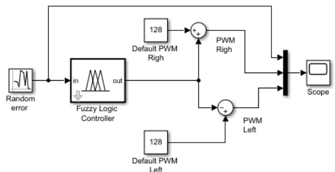
Gambar 8. Bagan Uji Fuzzy Logic Controller pada Matlab/Simulink
