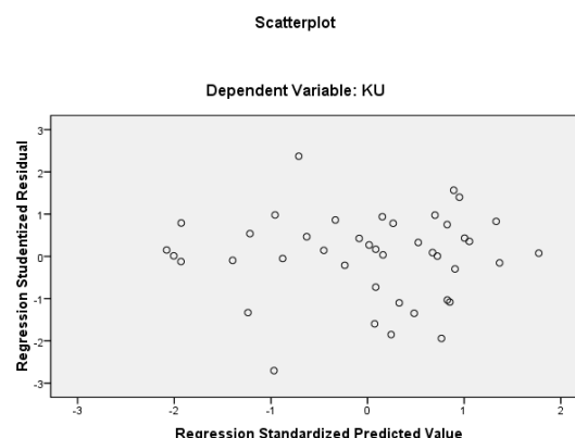
Gambar 2. Uji Heteroskedastisitas
