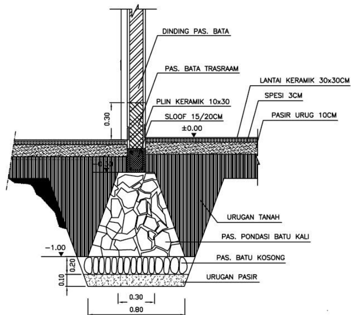
(a) (b) pasangan pondasi batu pada gambar 1.3 di bawah ini
