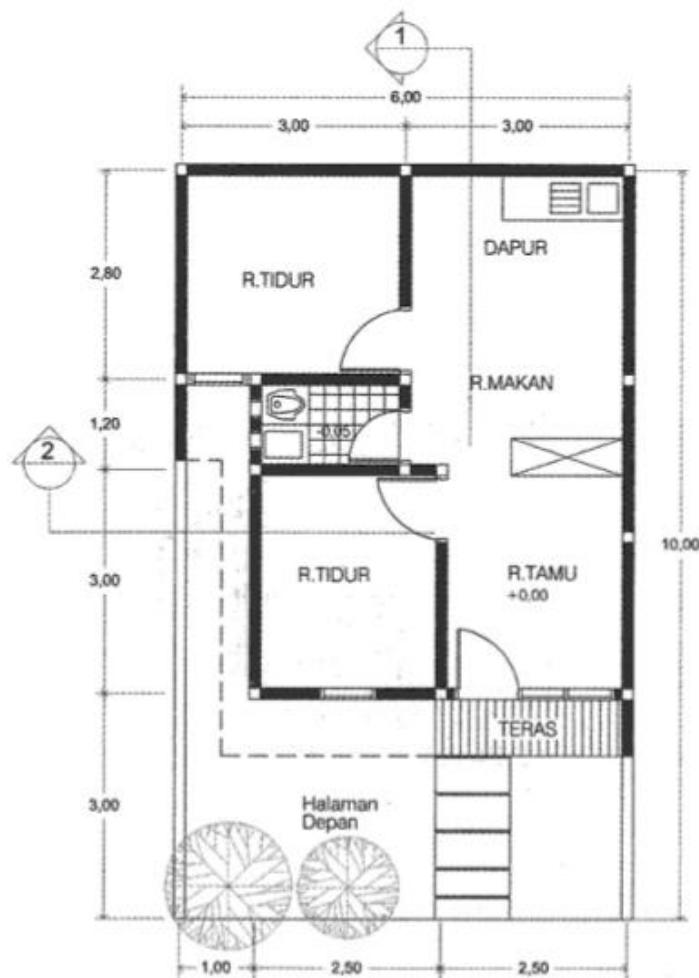
Gambar Rencana Desain Rumah
