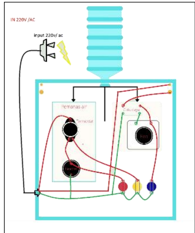
Gambar 1. Elemen-elemen dalam dispenser
