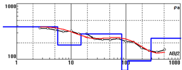
Gambar 6. Model Bawah Permukaan pada Titik 2
