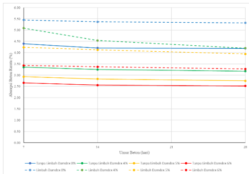
Gb. 8. Hubungan Absorpsi Beton dengan Umur Beton
