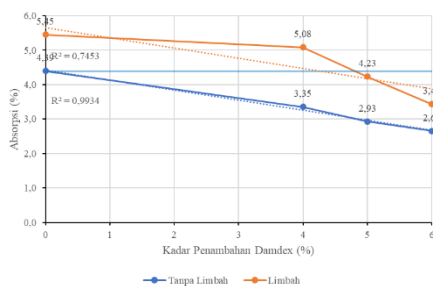
Gb. 5. Hubungan Absorpsi Beton dengan Kadar Penambahan Damdex pada Umur Beton 7 Hari
