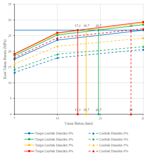
Gb. 4. Hubungan Kuat Tekan Beton dengan Umur Beton pada Berbagai Variasi Kadar Damdex
