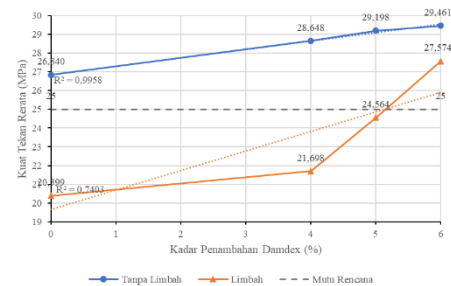
Gb. 2. Hubungan Kuat Tekan Beton dengan Kadar Penambahan Damdex pada Umur Beton 14 Hari
