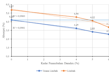
Gb. 6. Hubungan Absorpsi Beton dengan Kadar Penambahan Damdex pada Umur Beton 14 Hari
