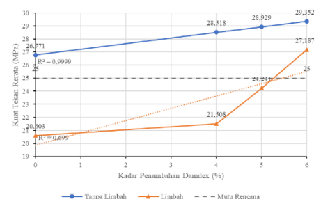
Gb. 3. Hubungan Kuat Tekan Beton dengan Kadar Penambahan Damdex pada Umur Beton 28 Hari
