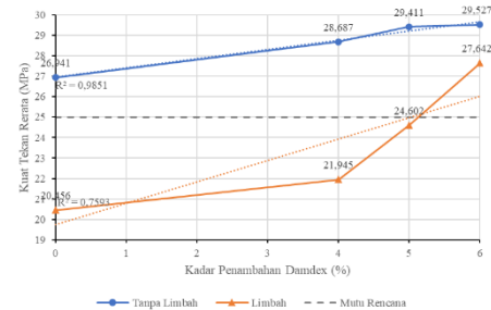
Gb. 1. Hubungan Kuat Tekan Beton dengan Kadar Penambahan Damdex pada Umur Beton 7 Hari
