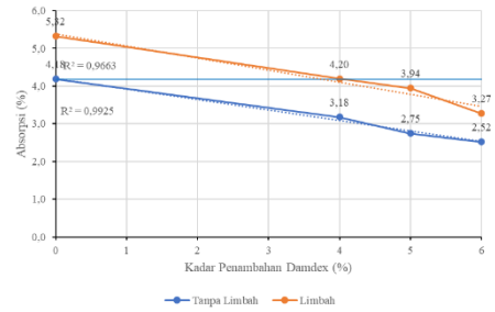
Gb. 7. Hubungan Absorpsi Beton dengan Kadar Penambahan Damdex pada Umur Beton 28 Hari
