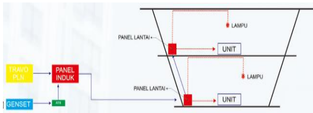
Gambar 11. Skema Jalur Listrik (Sumber: Analisa Penuli, 2024)
