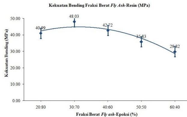
Gambar 6. Grafik kekuatan bending komposit Sumber: Dokumentasi Peneliti, 2023
