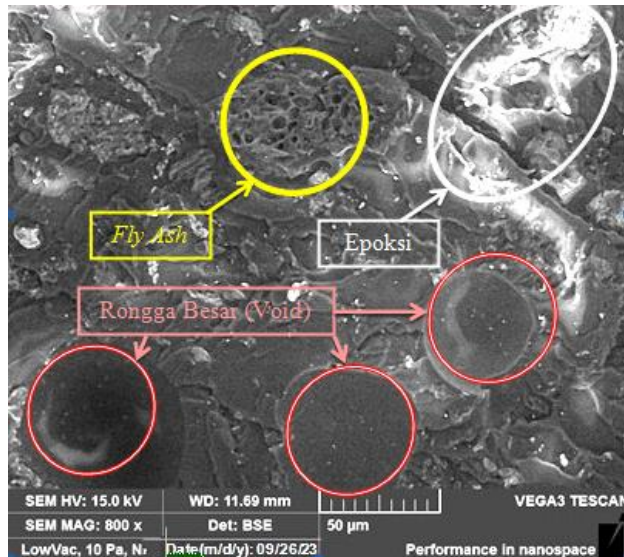
Gambar 7. Permukaan patah impact FB serbuk-matrik 60:40 Sumber: Dokumentasi Peneliti, 2023
