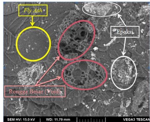
Gambar 8. Permukaan patah impact FB serbuk-matrik 40:60 Sumber: Dokumentasi Peneliti, 2023.
