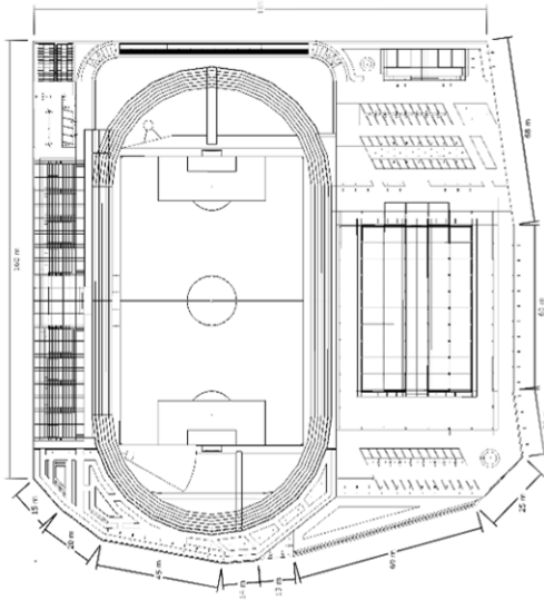
Gambar 7. Layoutplan (Sumber: Penulis)
