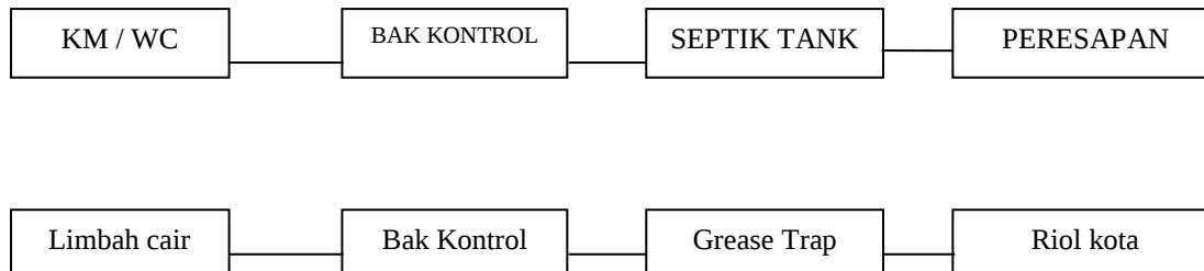
Gambar 3. Jaringan Sanitasi
