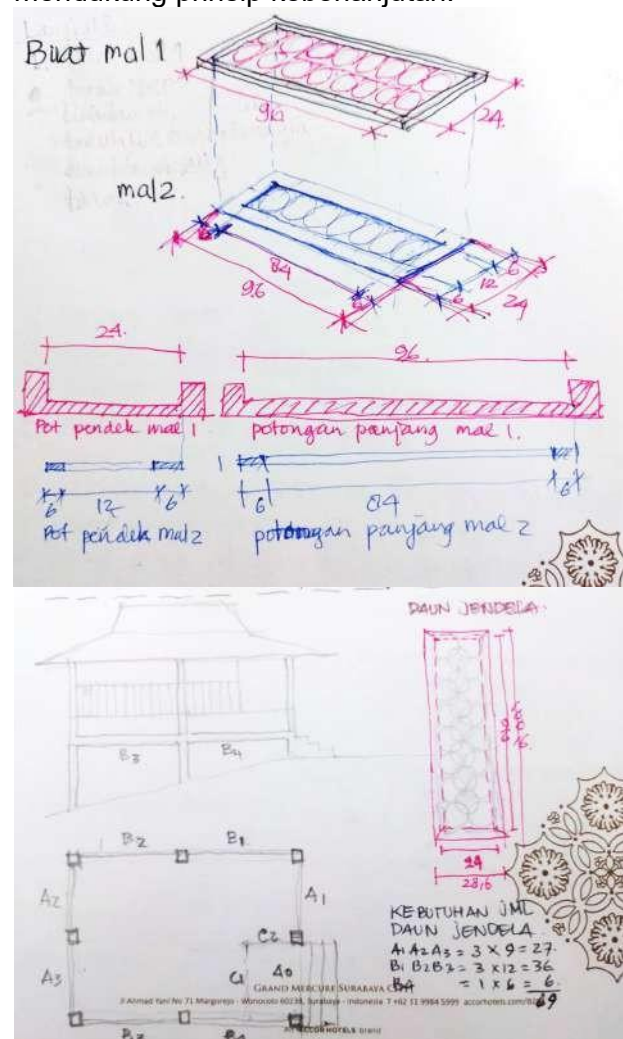
Gambar 4. Sketsa awal lontaran desain (Sumber: Dokumentasi Penulis, 2023)
