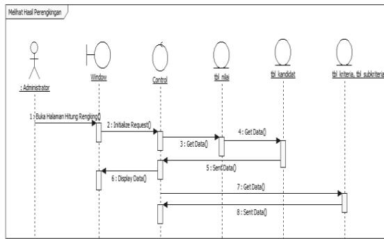
Gambar 6 : Sequence diagram melihat hasil perangkingan
