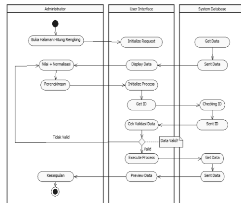
Gambar 4: Hasil Perangkingan
