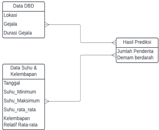
Gambar 3 Rancangan DB
