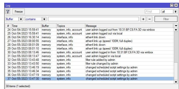
Gambar 27. Log Mikrotik
