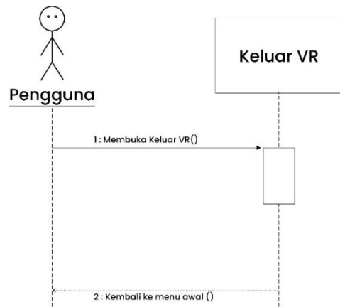
Gambar 8 Sequence Diagram Menu Keluar VR
