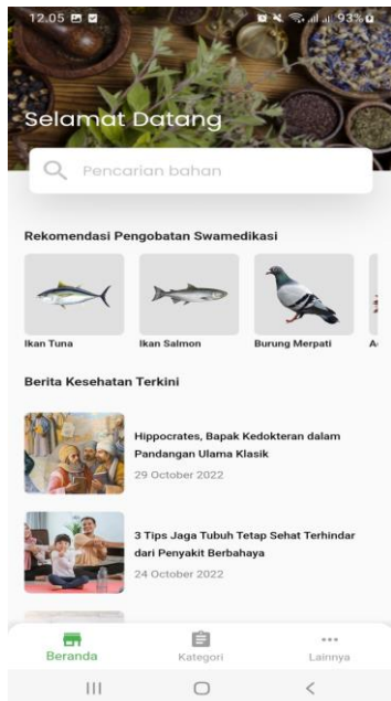
Gambar 3. Halaman beranda
