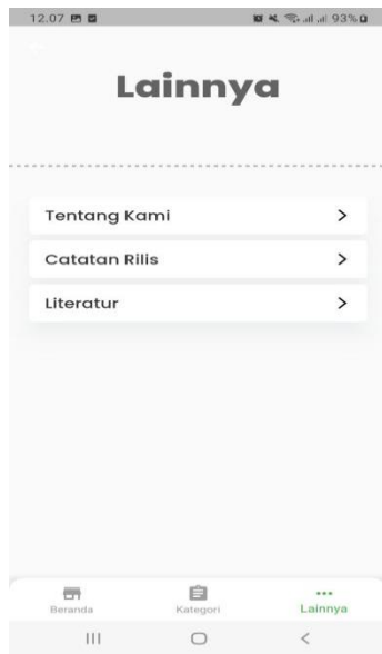
Gambar 10. Halaman lainnya
