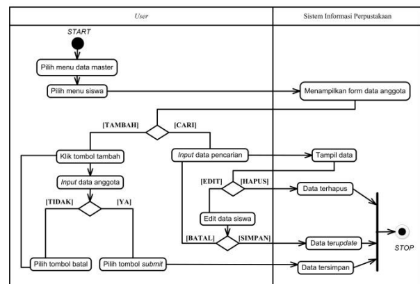
Gambar 5 Activity Diagram Tambah Anggota
